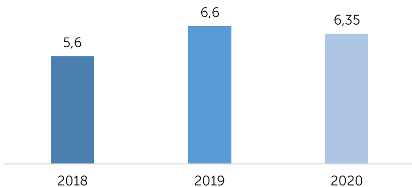
Caudal (m 3 /s) tratado por la PTAR-C en Cali (2018-2020).
