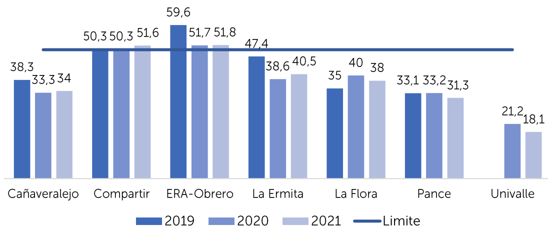
Niveles de PM 10 (µg/m 3 ) en las estaciones del DAGMA en Cali (2019-2021). *
