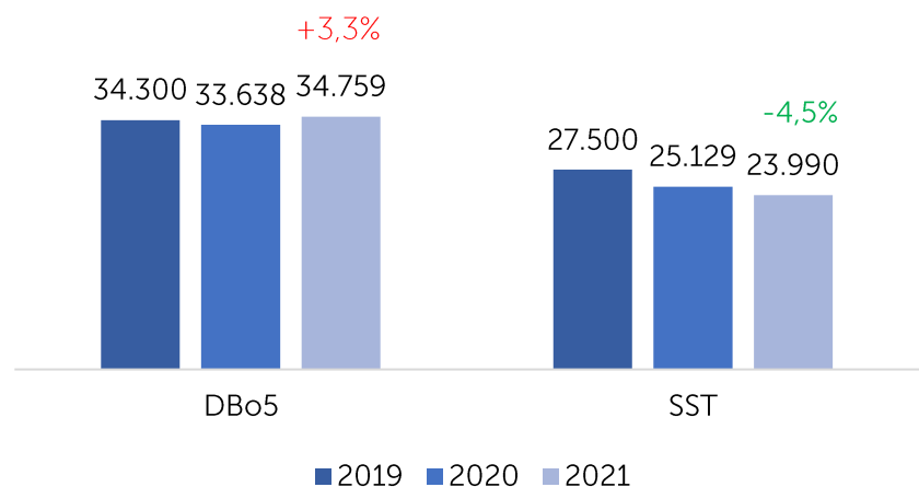
Cargas contaminantes vertidas en el Río Cauca (2019 -2021) (Cifras en toneladas).
