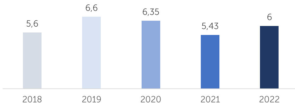
Caudal (m 3 /s) tratado por la PTAR-C en Cali (2018-2022)
