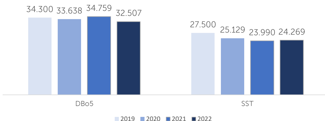
Cargas contaminantes vertidas en el Río Cauca (2019 -2022) (Cifras en toneladas)
